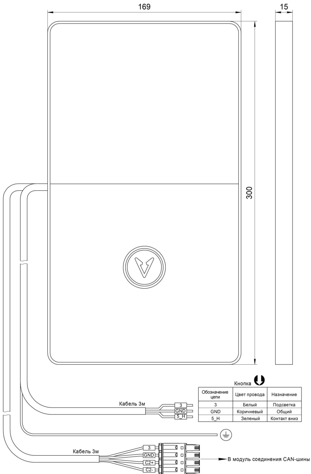
Рис.1 Внешний вид Вызывной пост ОНИКС НШЕК.468381.023-01
